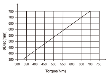
扭力曲線表
