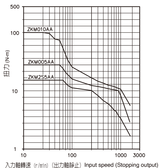
【容許滑動扭力特性圖】 Allowable slipping torque chart
