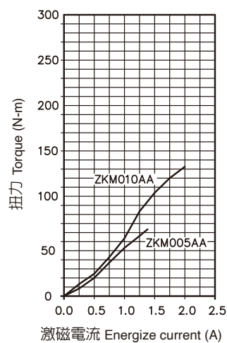
【容許滑動扭力特性圖】 Allowable slipping torque chart
