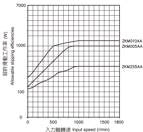
【容許滑動功率特性圖】 Allowable slipping efficiency chart
